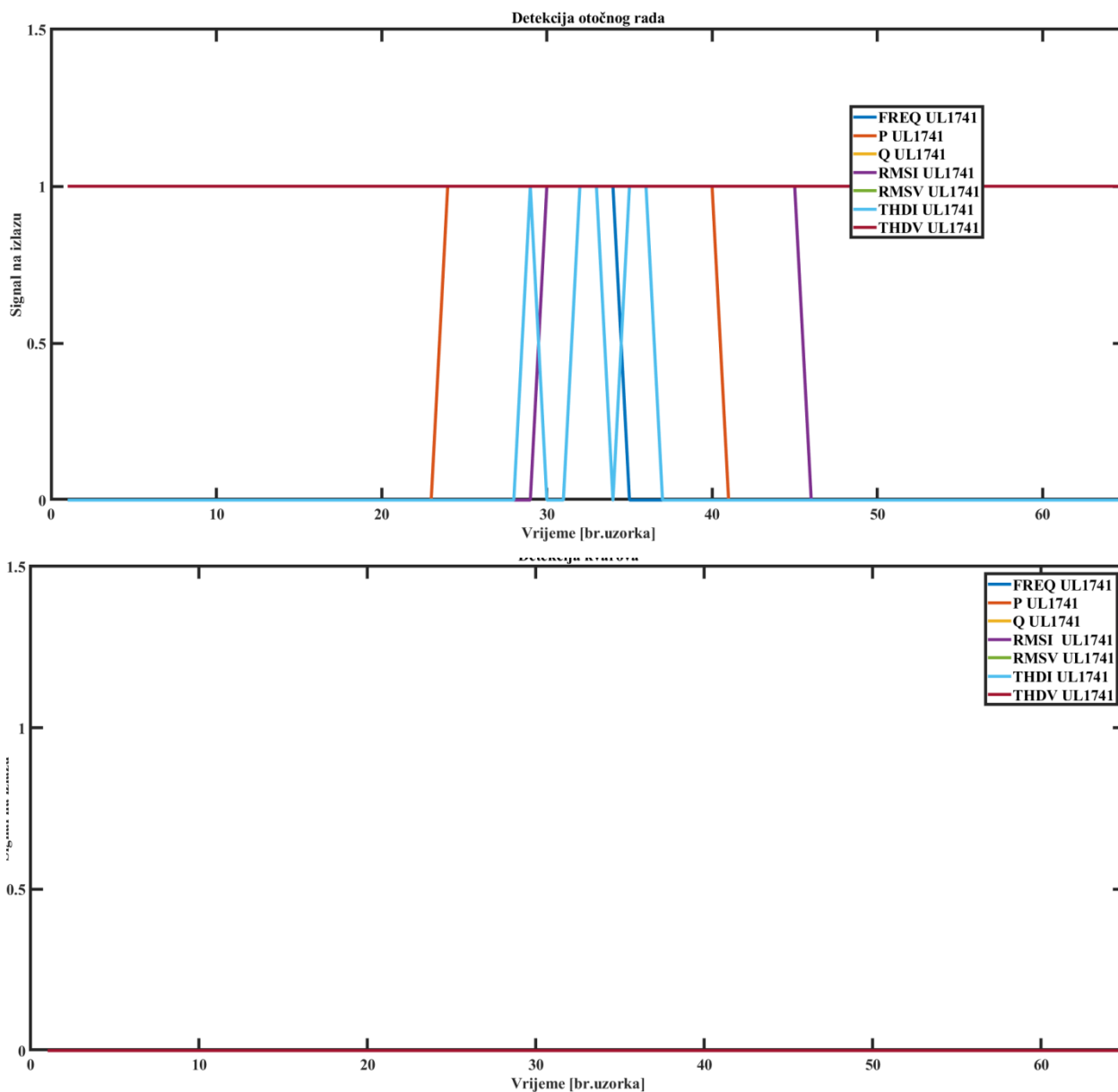
Slika 8.18. Rezultati testiranja MPV metode pri standardu UL1741. Pod uvjetima različitih faktora kvalitete mreže se vidi da MPV prepoznaje prelazak u otočni rad dok MPV dežurna za kvarove se ne aktivira.
