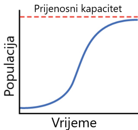
Slika 5.1. Logistički rast populacije
