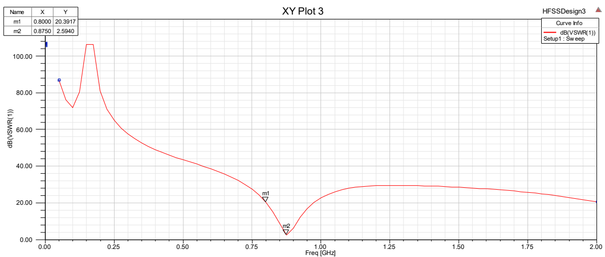
4.2.1.9. slika VSWR parametra metamaterijalne antene
