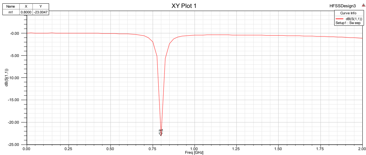
4.2.2.11. slika S_{11} parametra metamaterijalne antene
