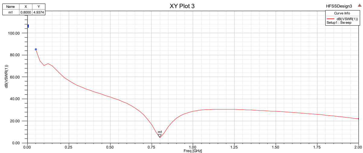
4.2.3.6. slika VSWR parametra metamaterijalne antene
