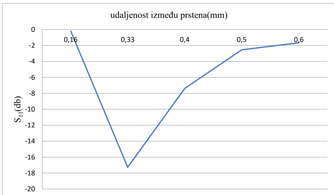
4.2.1.1. grafikon ovisnosti parametra S_{11} o duljini razmaka između prstena
