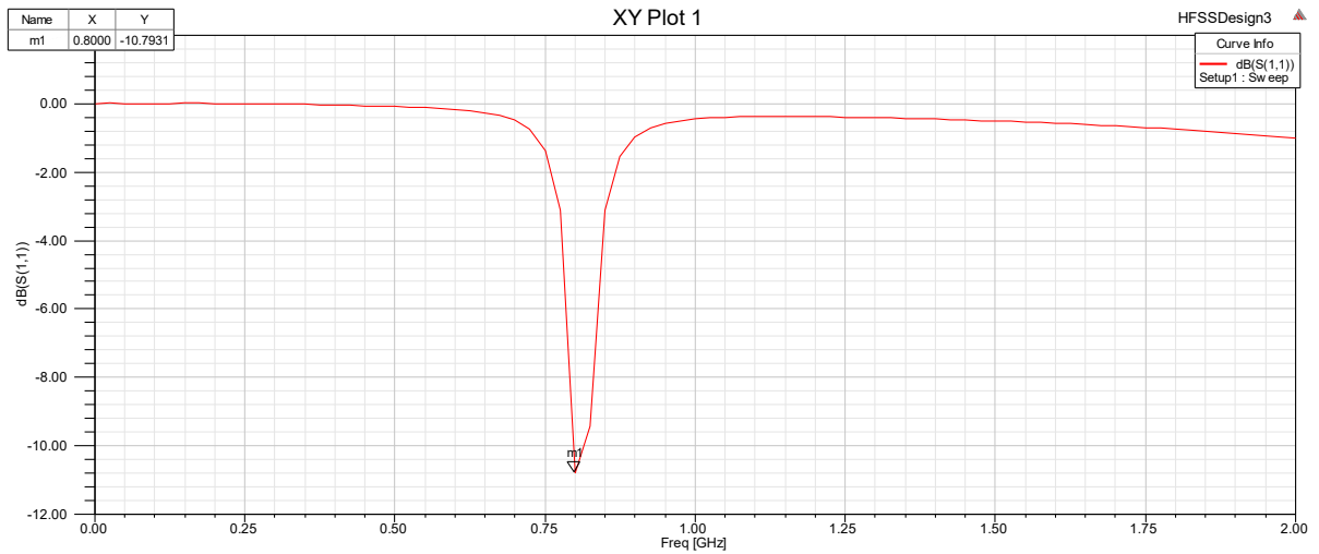
4.2.2.15. slika S_{11} parametra metamaterijalne antene
