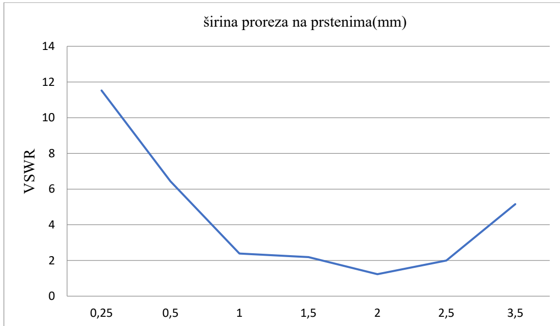
4.2.2.2. grafikon ovisnosti VSWR o širini proreza
