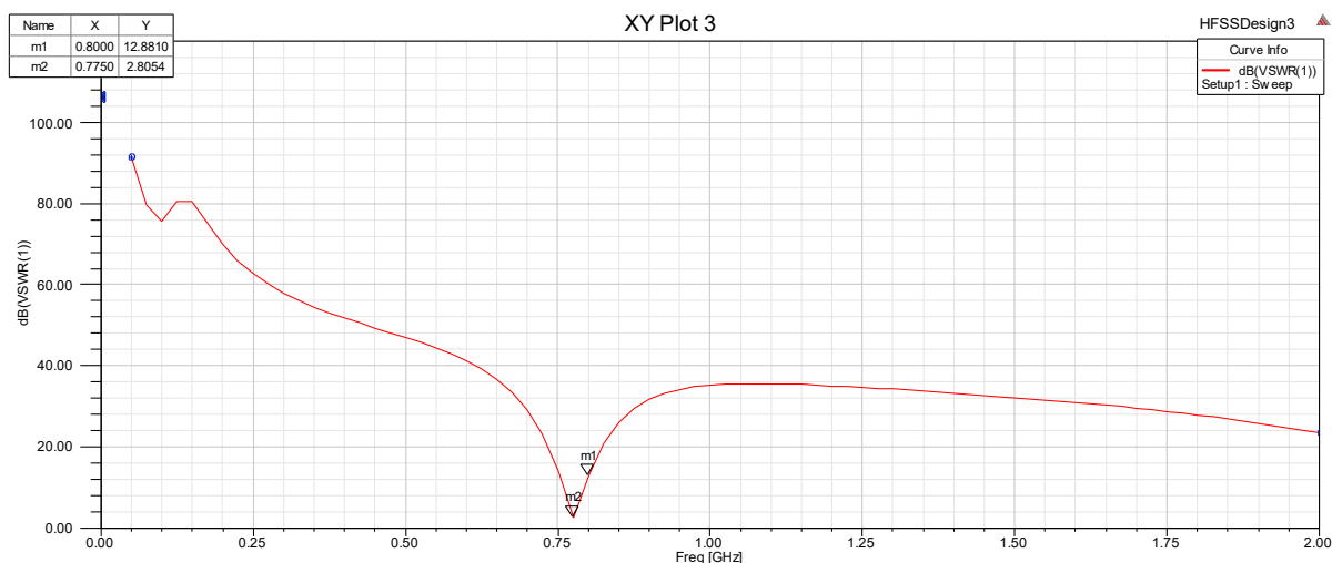
4.2.3.14. slika VSWR parametra metamaterijalne antene
