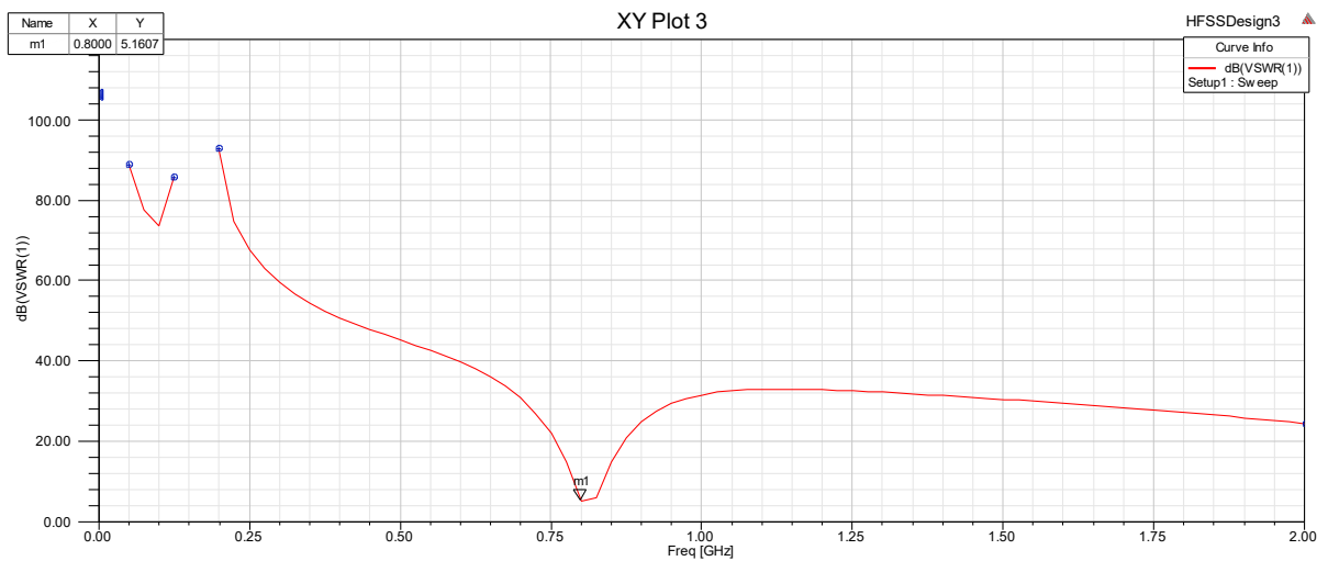
4.2.2.16. slika VSWR parametra metamaterijalne antene
