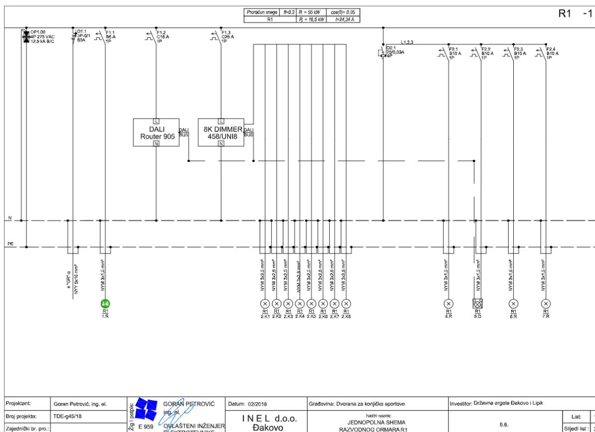
Sl. 5.1.2. Jednopolna shema razvodnog ormara R1 s Državne ergele Đakovo i Lipik [21]
