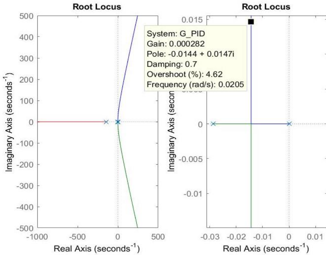
Slika 4.2. Krivulja mjesta korijena kompenziranog procesa 3. reda lijevo i поблиzi pogled na dominantne polove desno
