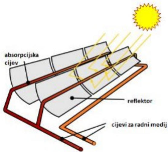
Slika 3.5. Jednostavni prikaz funkcioniranja paraboličnog žljebastog kolektora [5]
