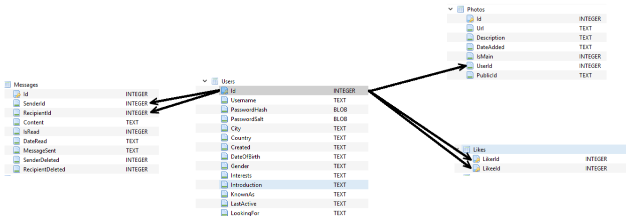
Slika 4.3 Dijagram baze podataka
