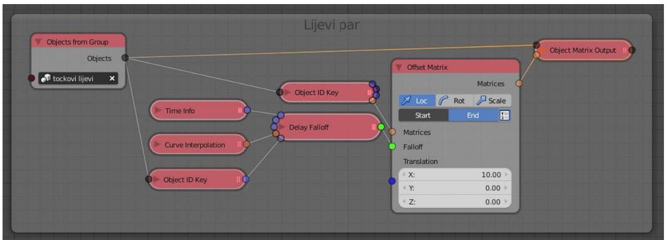
Slika 4.8. Stablo čvorova za lijevi par kotača
