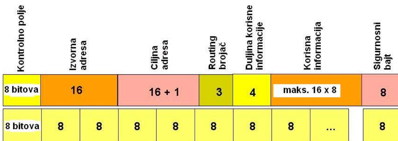
Slika 3.8. Struktura telegrama [5]
