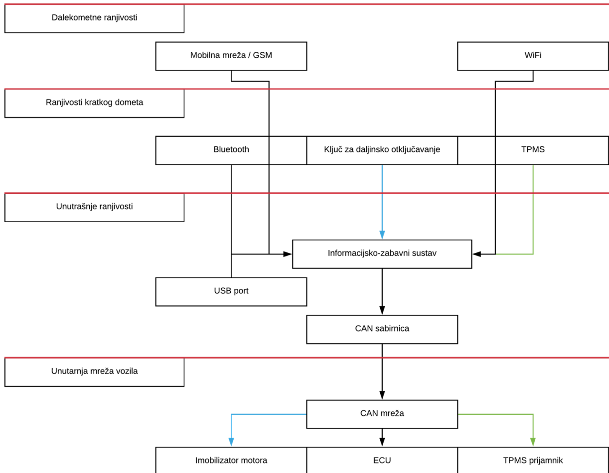
Slika 2.1. Prikaz arhitekture prijamnika u automobilu
