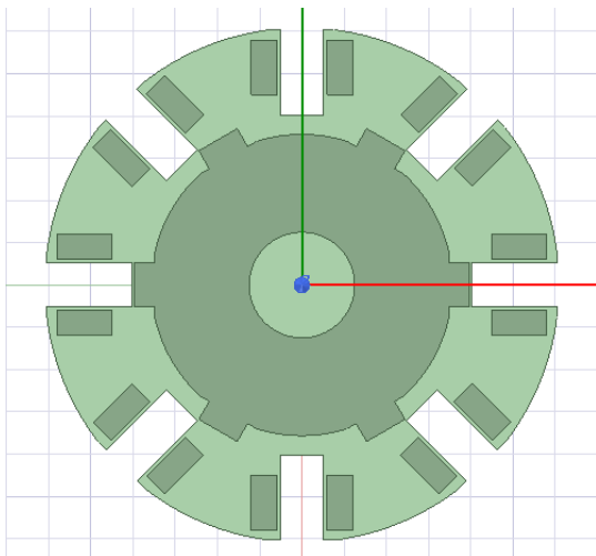
Slika 4.10. Unutrašnjost statora (rotor i namoti)
