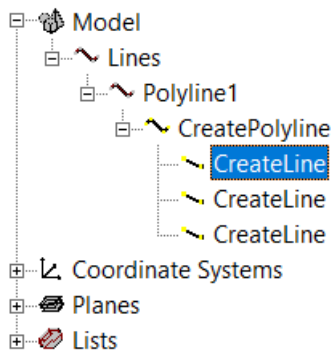
Slika 4.3. Izbornik „Model“
