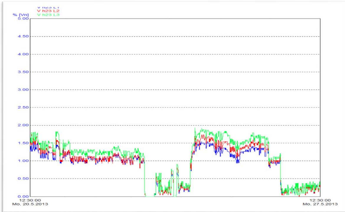
Slika 4.5. Prikaz 23. harmonika
