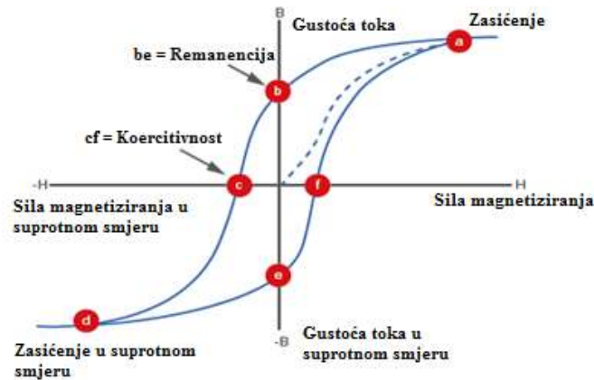
Slika 3.5. Petlja histereze.
