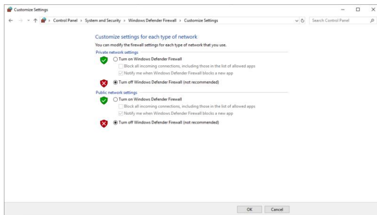
Slika 7.1. – Windows Firewall
