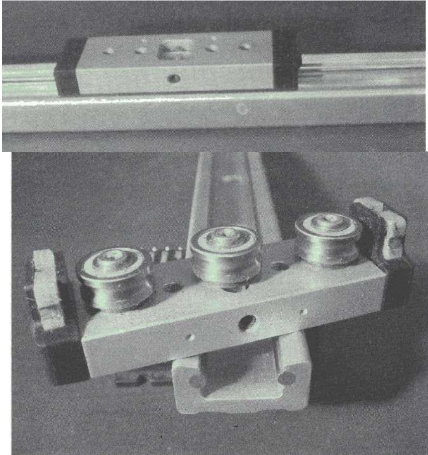
Slika 2.9: sustav hibridne valjčane vodilice
