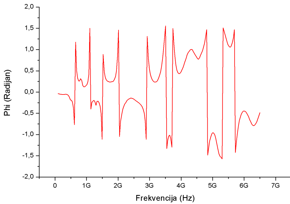
Slika 7.20. Fazni kut
