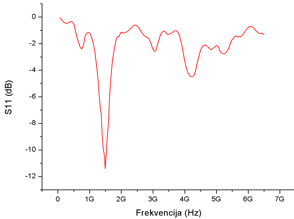
Slika 8.12. S11 Parametar
