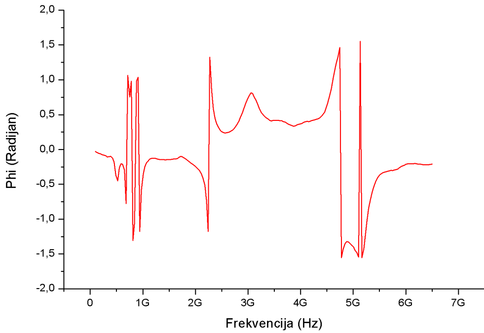
Slika 7.10. Fazni kut
