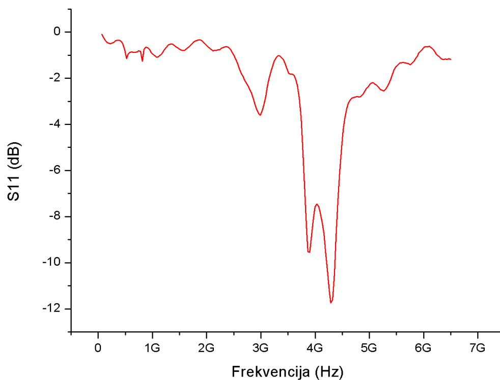
Slika 8.17. S11 Parametar
