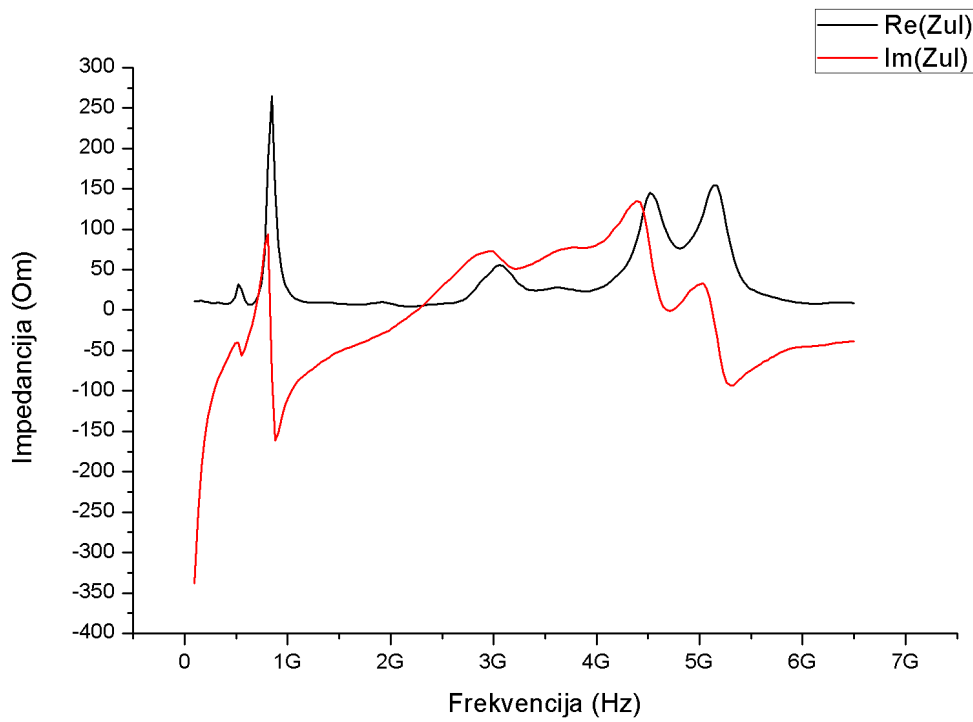
Slika 7.3. Realni i imaginarni dio impedancije
