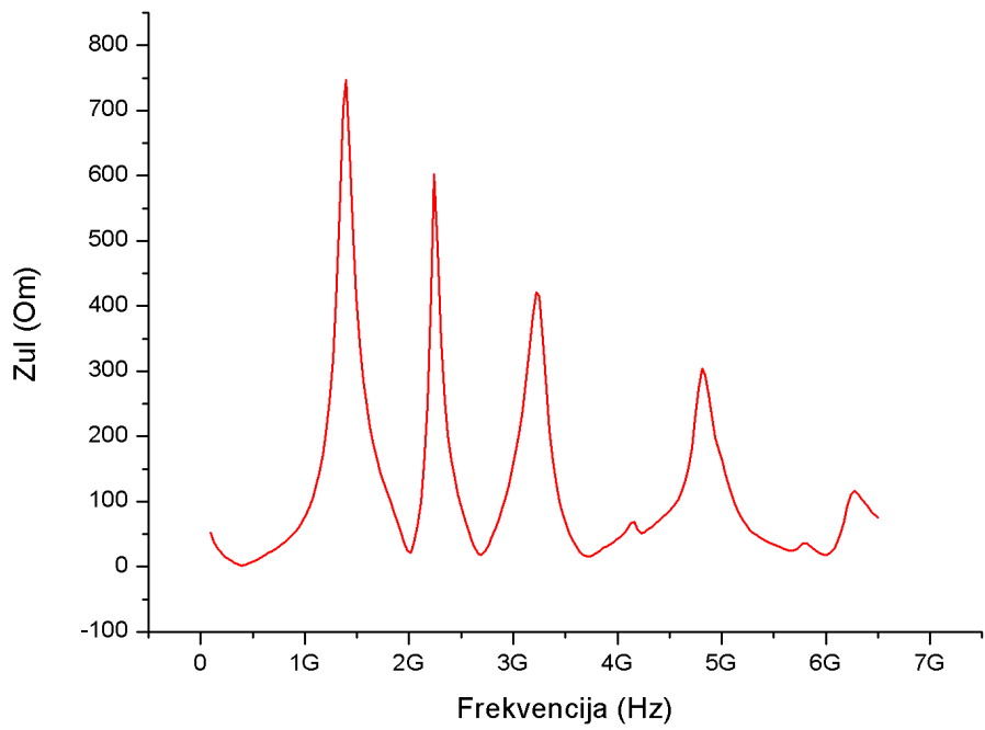
Slika 5.29. Ulazna impedancija
