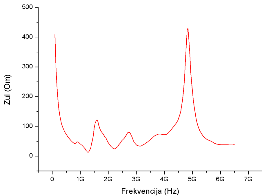
Slika 8.4. Ulazna impedancija
