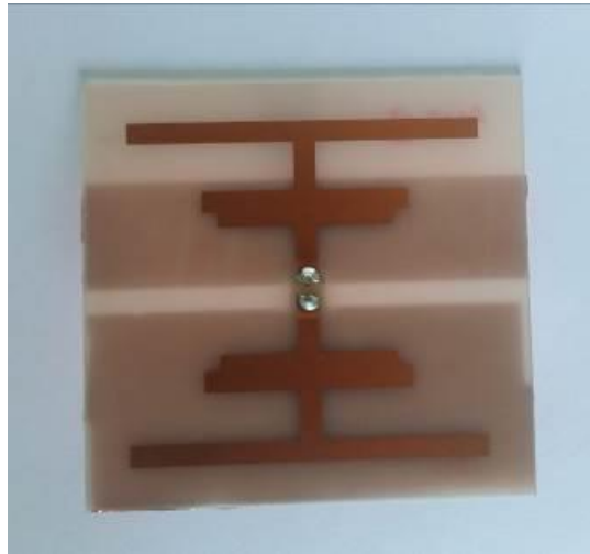
Slika 3.16. Tip-1 s tri bakarne trake
