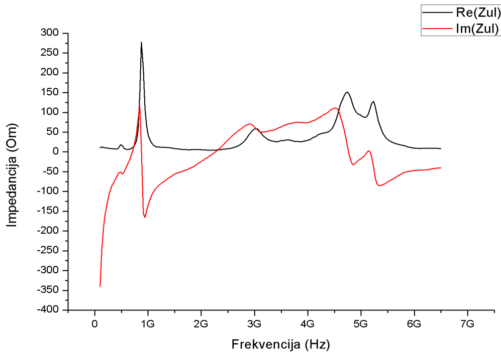
Slika 7.13. Realni i imaginarni dio impedancije
