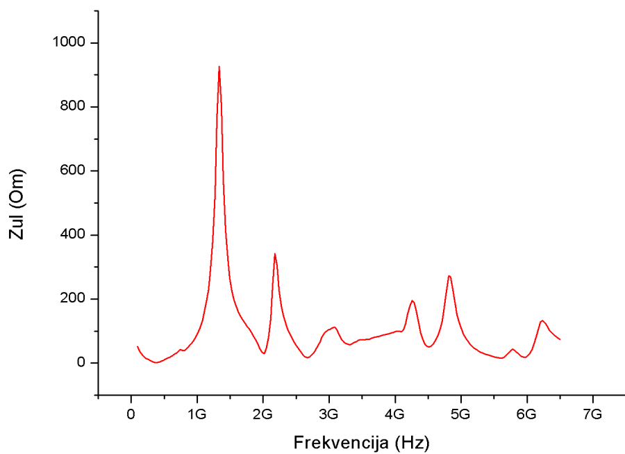
Slika 5.24. Ulazna impedancija
