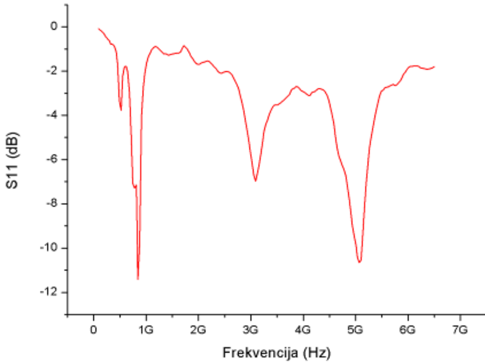
Slika 7.2. S11 Parametar
