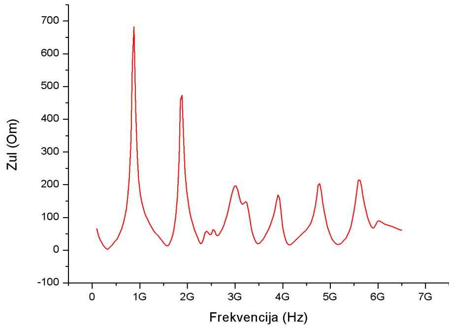
Slika 7.29. Ulazna impedancija
