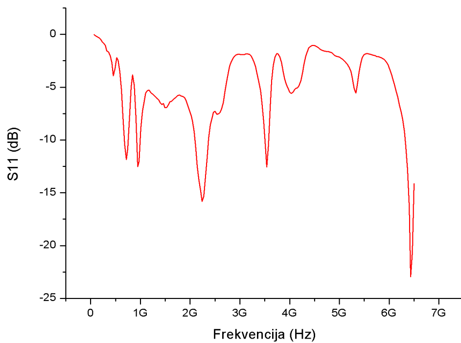
Slika 6.22. S11 Parametar
