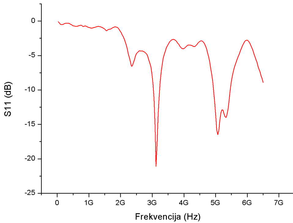
Slika 3.17. S11 Parametar
