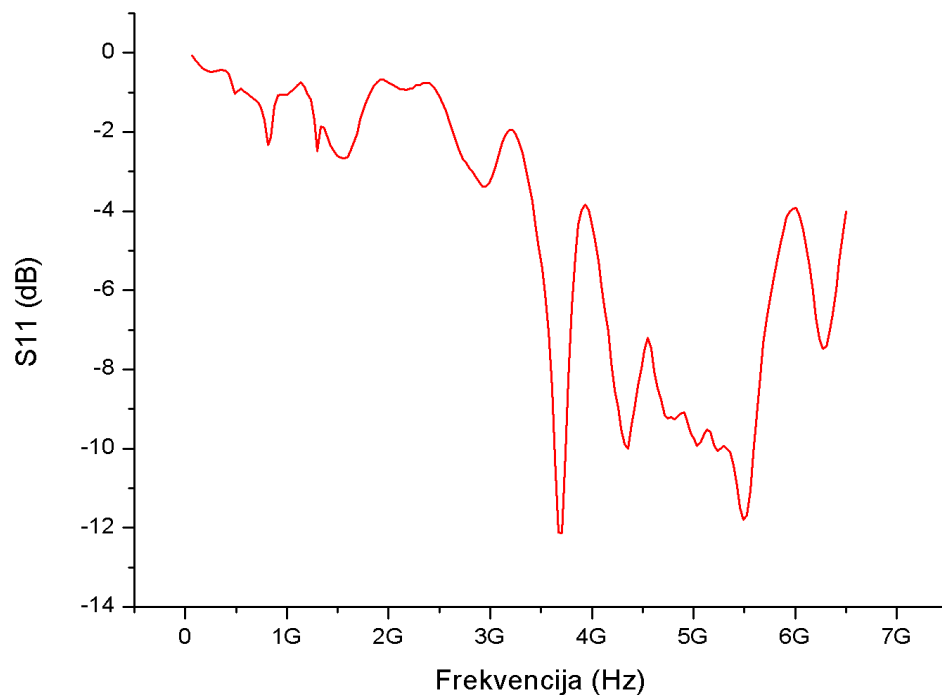
Slika 7.17. S11 Parametar
