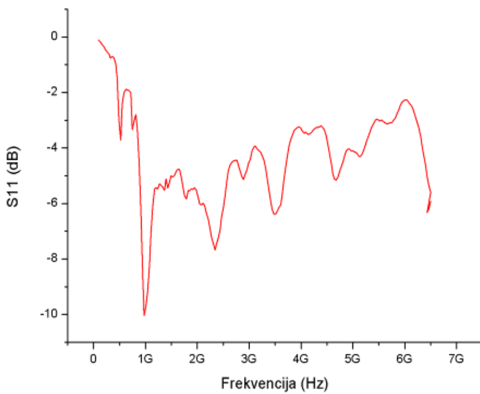
Slika 3.7. S11 Parametat
