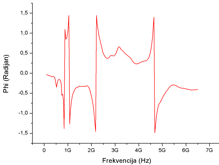
Slika 5.10. Fazni kut
