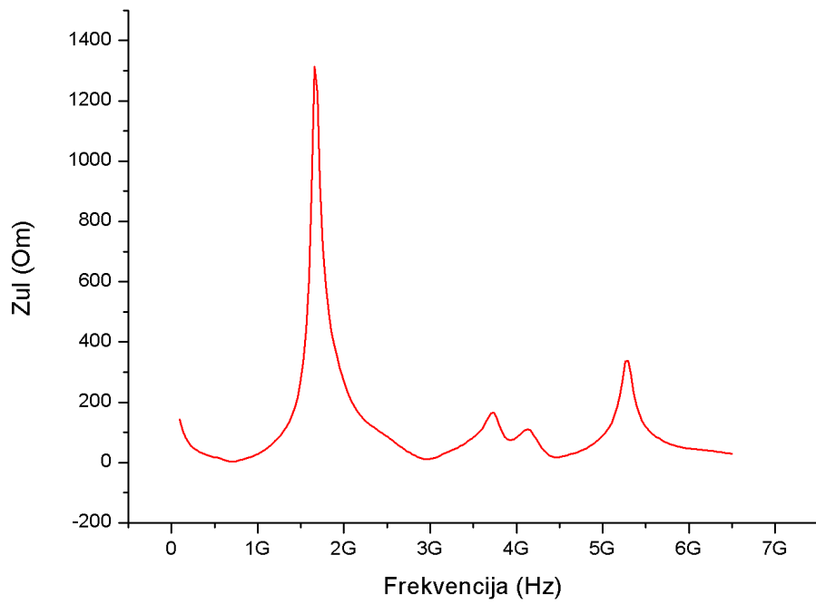
Slika 8.19. Ulazna impedancija
