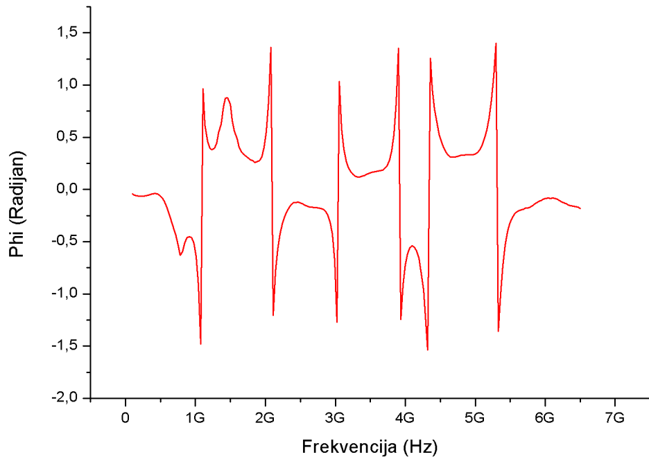
Slika 8.10. Fazni kut
