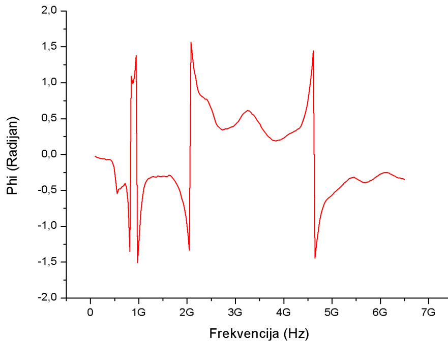
Slika 5.5. Fazni kut
