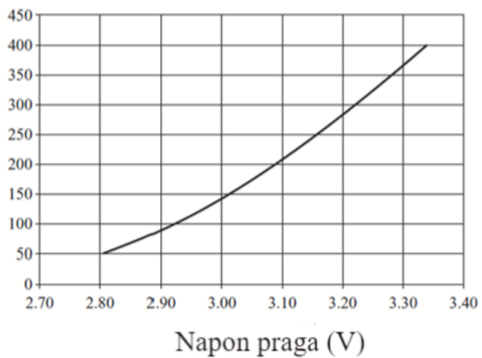
Slika 3. 4. Napon praga kao funkcija struje [2].
