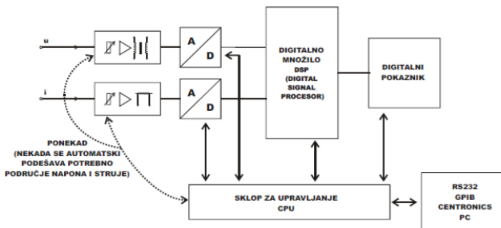
Slika 3.2 - Digitalni vatmetar [3]
