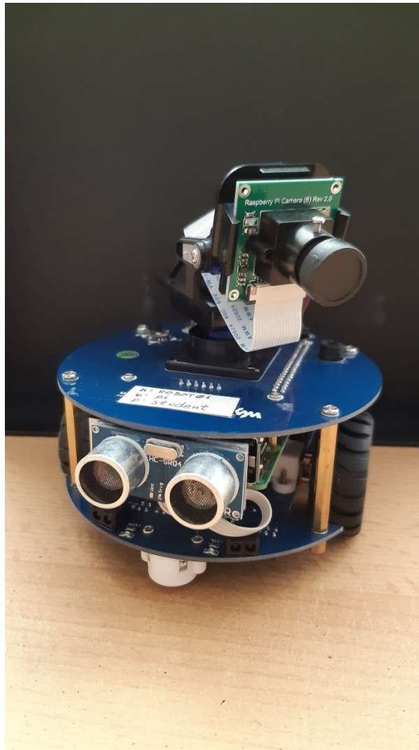
Slika 2.1 AlphaBot2 PI
