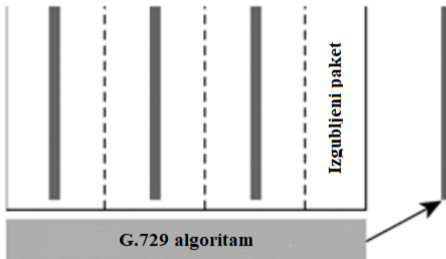
Sl.2.5. Mehanizam ponavljanja posljednjeg primljenog paketa [1]
