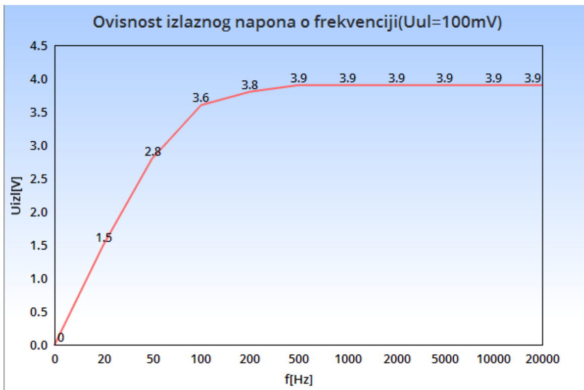
Slika 4.9. Ovisnost izlaznog napona o frekvenciji pri ulaznom naponu U ul =100mV
