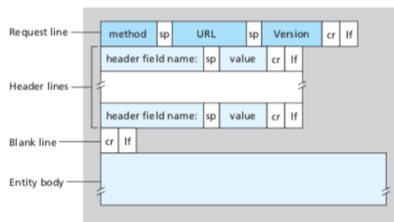
Slika 3.2. Poopćeni format HTTP zahtjeva
