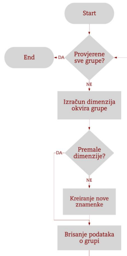
Slika 3.6.: Dijagram toka Labels2Digits() funkcije.
