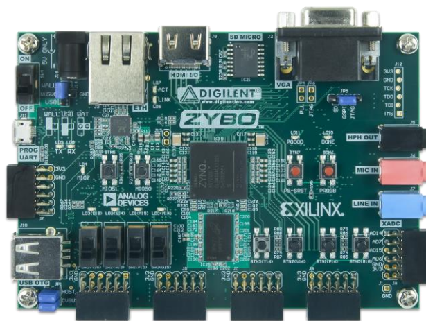
Slika 2.13.: ZYBO platforma. [16]
