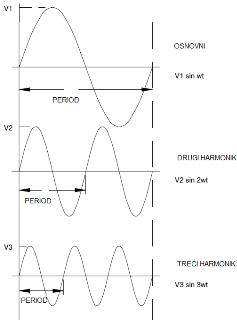
Slika (3.4.) Osnovni, drugi i treći harmonik [9]
