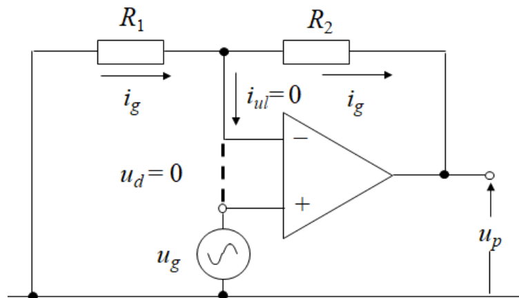
Slika 3.5. Ne-invertirajuće pojačalo [9]
