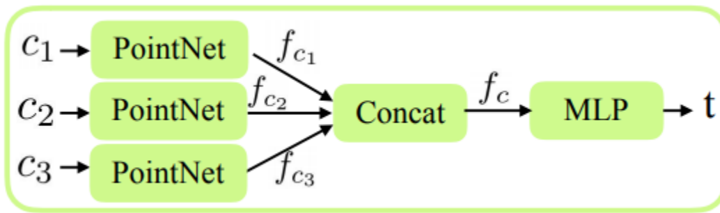
Slika 3.2. Grafički prikaz arhitekture Mreže predviđanja središta
