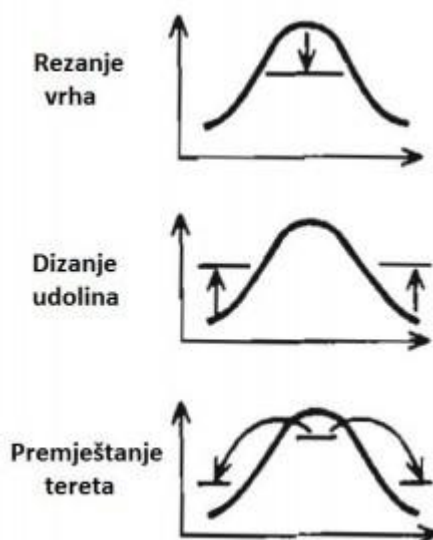
Slika 4.1. Ciljevi modifikacija krivulje opterećenja [4]
