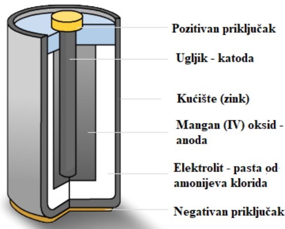
Slika 4.1. Prikaz presjeka strukture cink-ugljik baterije [14]
