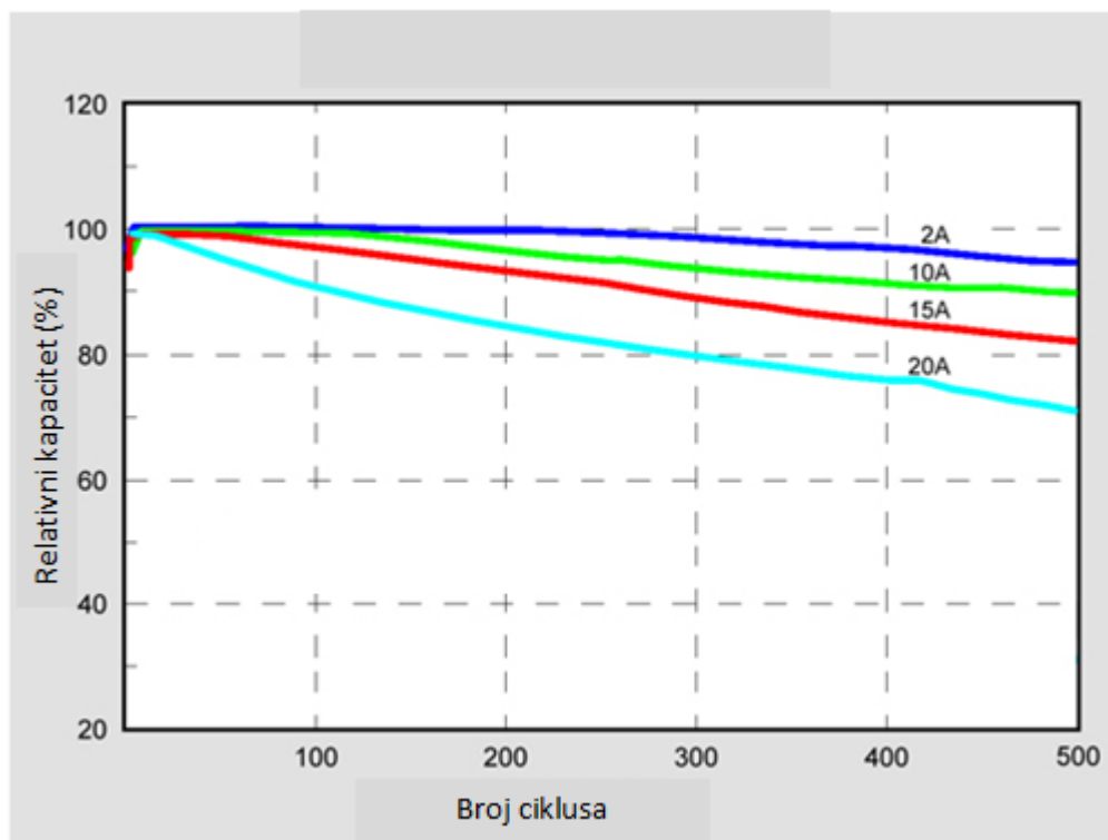
Slika 3.6. Ovisnost kapaciteta i broja ciklusa o struji pražnjenja
