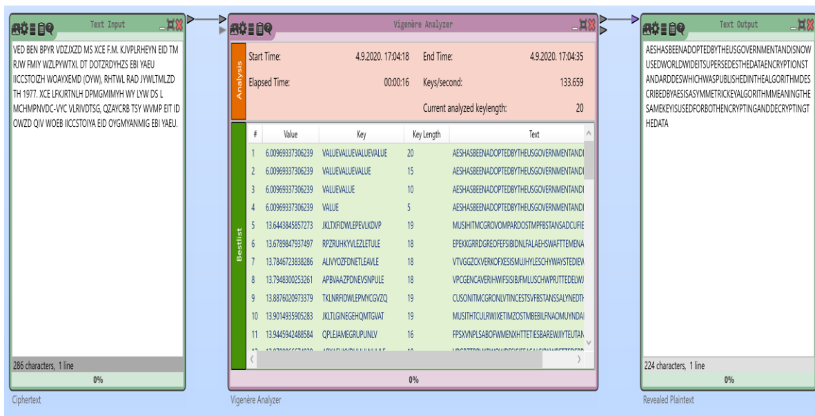
Slika 5.20 Primjer 3: Vigenerova analiza
