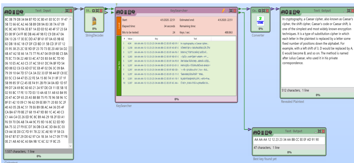
Slika 5.27 Primjer 5: AES analiza korištenjem entropije
