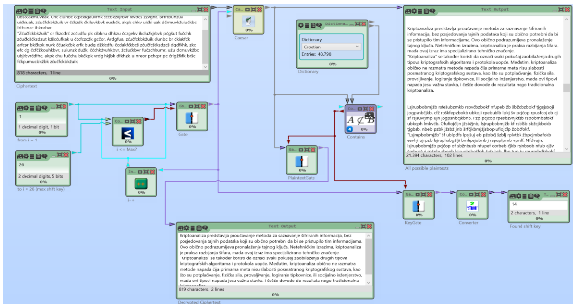
Slika 5.15 Primjer 4: Kriptoanaliza Cezarove šifre „grubom silom“
