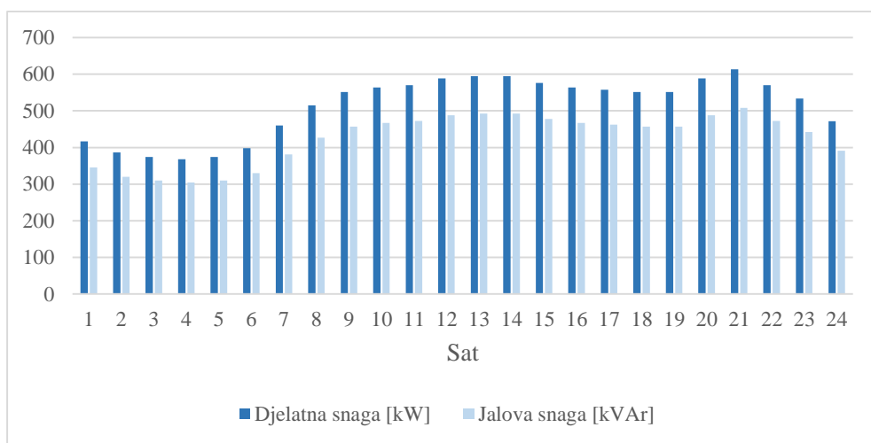
Slika 5.6. Dijagram opterećenja koji prikazuje vrijednosti djelatne i jalove sage za sabirnicu 9
