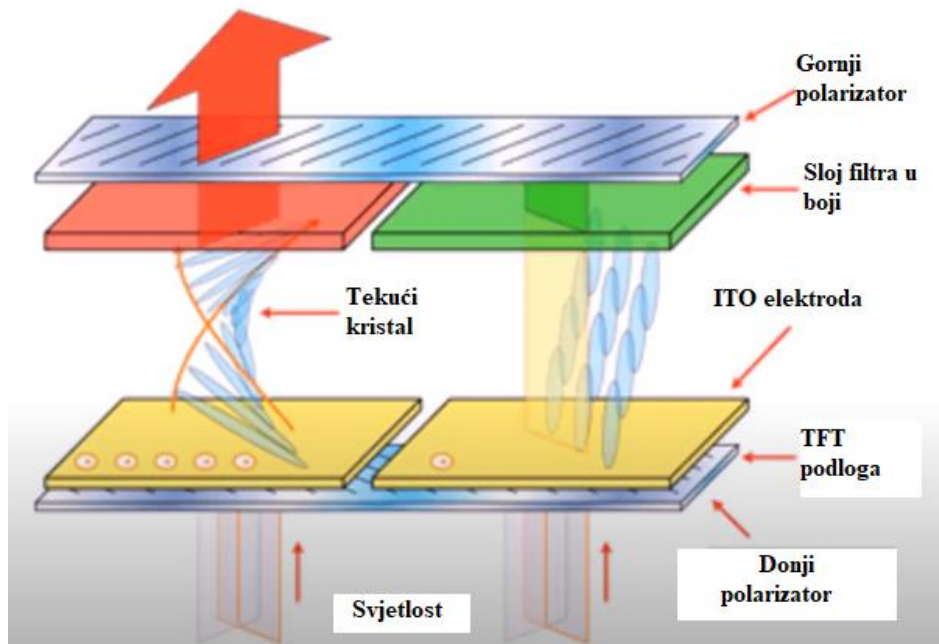
Slika 3.12. – Prikaz zadaće tranzistora u funkciji LCD televizora, [17].
