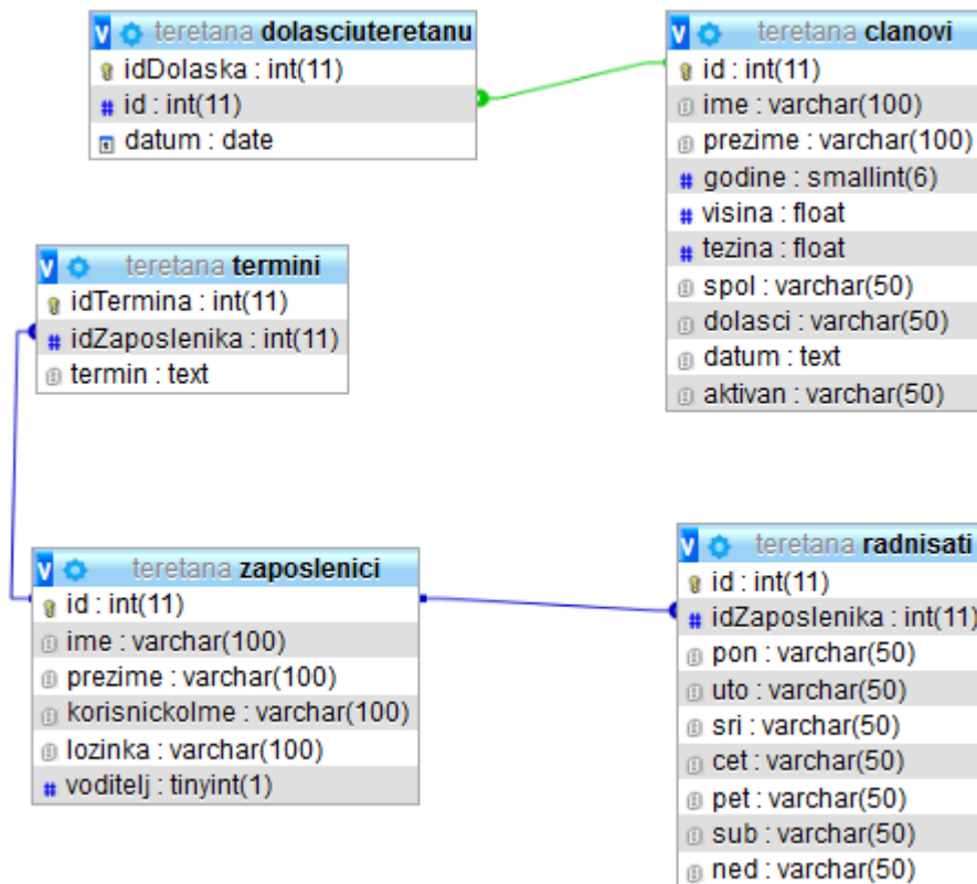
Slika 3.6. E-R dijagram baze podataka.
