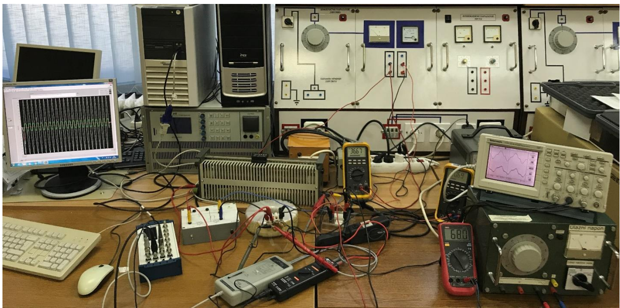
Slika 3.2. Laboratorijski sustav.
