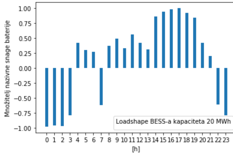
Slika 8.15: Krivulja punjenja i pražnjenja BESS-a kapaciteta 20 MWh
