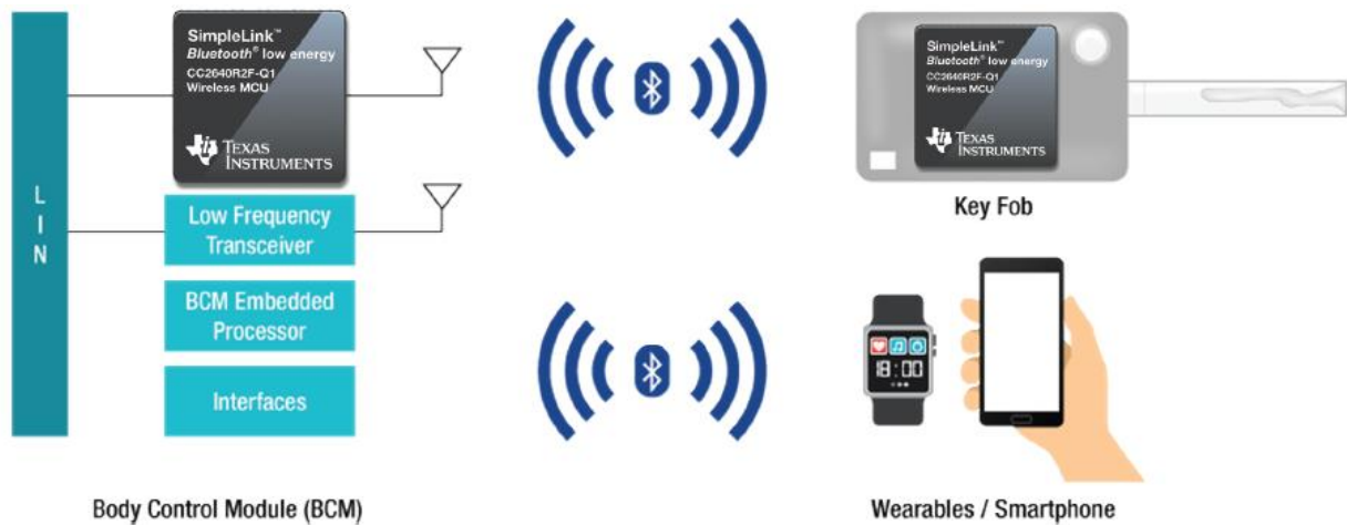
Slika 4.1. Blok dijagram pristupa automobilu korištenjem BLE aplikacije [25]
