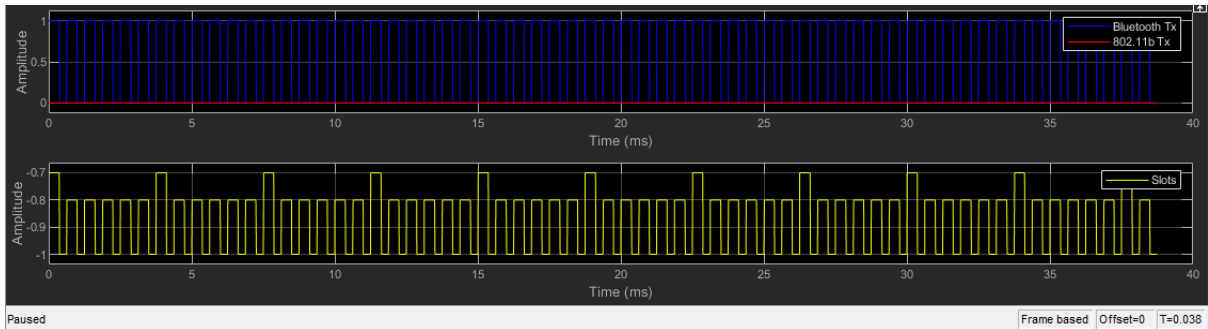
Slika 5.40. Vremenski dijagram primljenog signala DM1/AWGN/1&2
