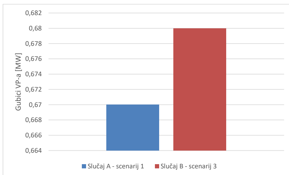
Slika 6.19. Gubici VP-a pri varijanti 1
