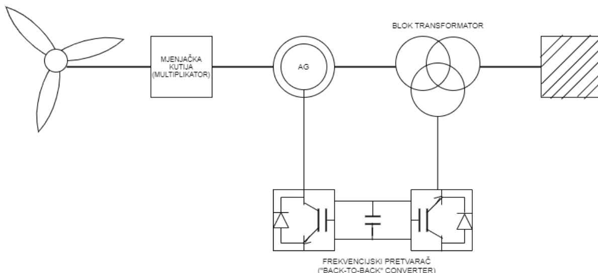
Slika 3.1. Vjetroagregat Tip 3 [12]
