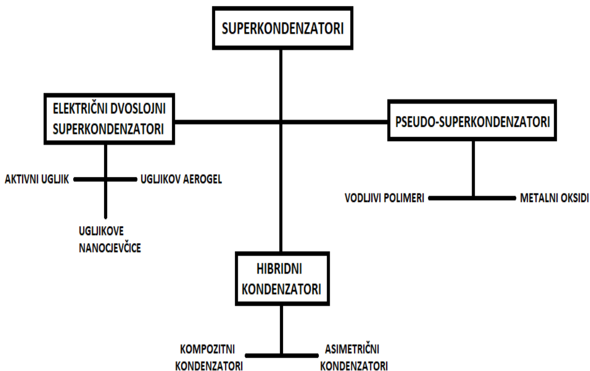
Slika 4.1. Podjela superkondenzatora
