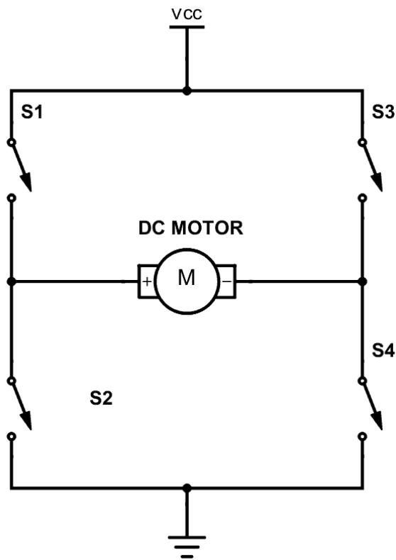
Slika 2.9. spoj H-most [7]
