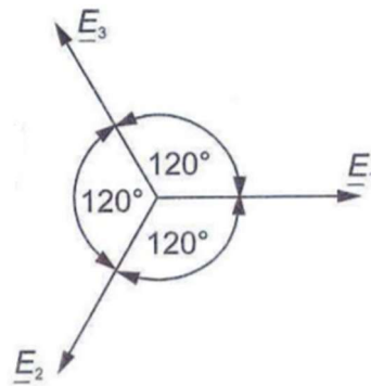
Slika 3.6 Naponi trofaznog generatora prikazano kao tri rotirajuća fazora ( E_1, E_2, E_3 -efektivne vrijednosti induciranog napona ) [10]
