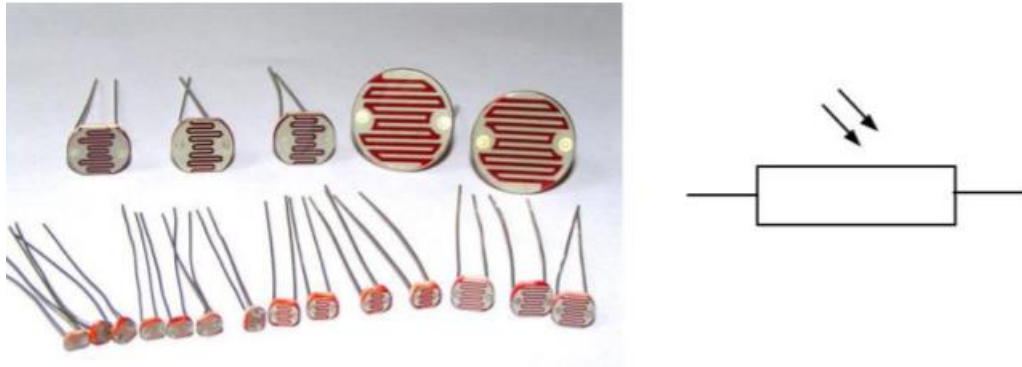
Slika 4.10. Prikaz LDR otpornika i simbol (IEC standard)
