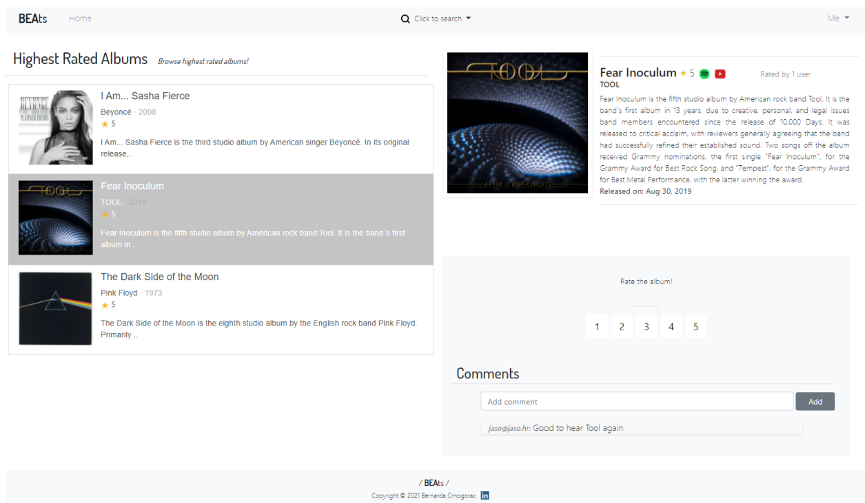
Slika 4.12. Album-detail-highest komponenta
