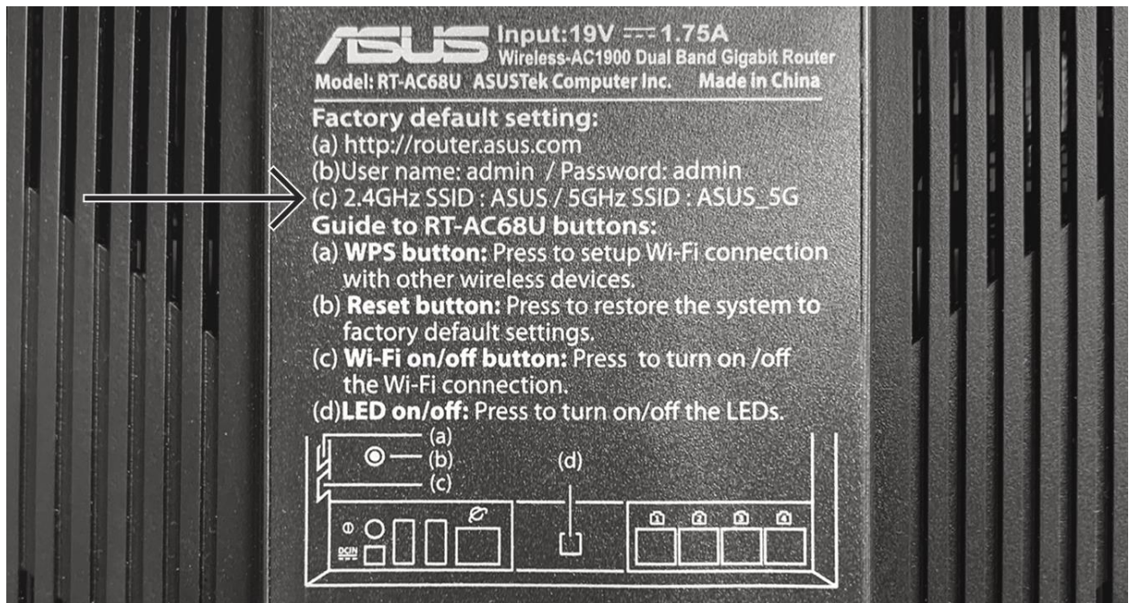
Slika 3.2. Prikaz pretpostavljenog SSID-a na usmjerivaču [9]
