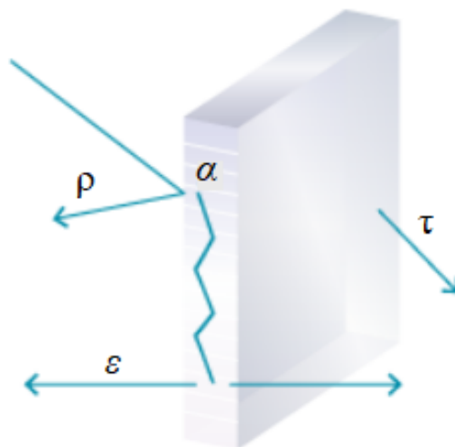
Slika 2.6. Karakteristike zračenja tijela
