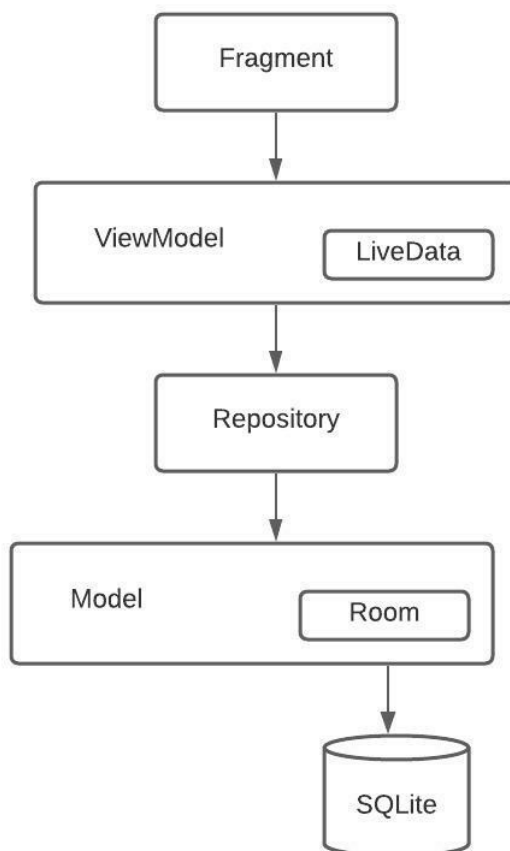
Slika 4.1. Arhitektura aplikacije
