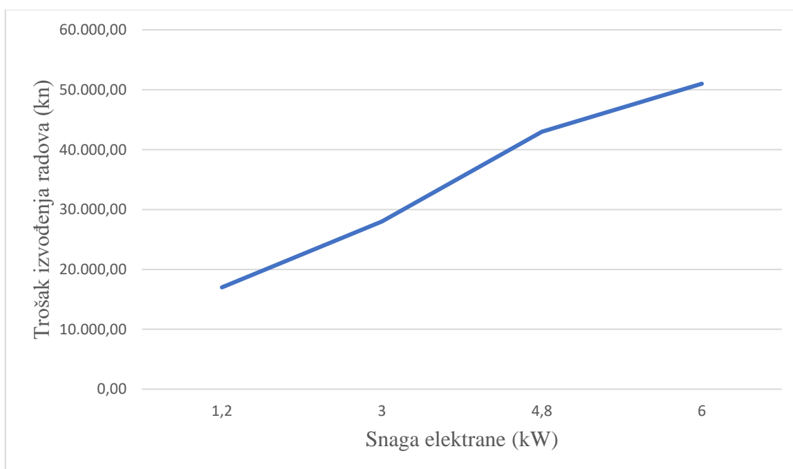
Slika 3.27. Trošak ugradnje fotonaponske elektrane u ovisnosti o snazi.
