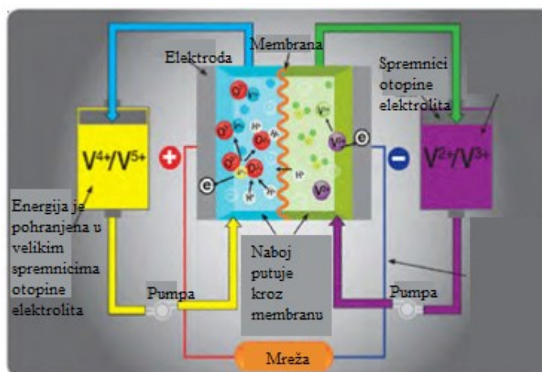
Slika 4.5. Shematski prikaz protočne baterije, [11].
