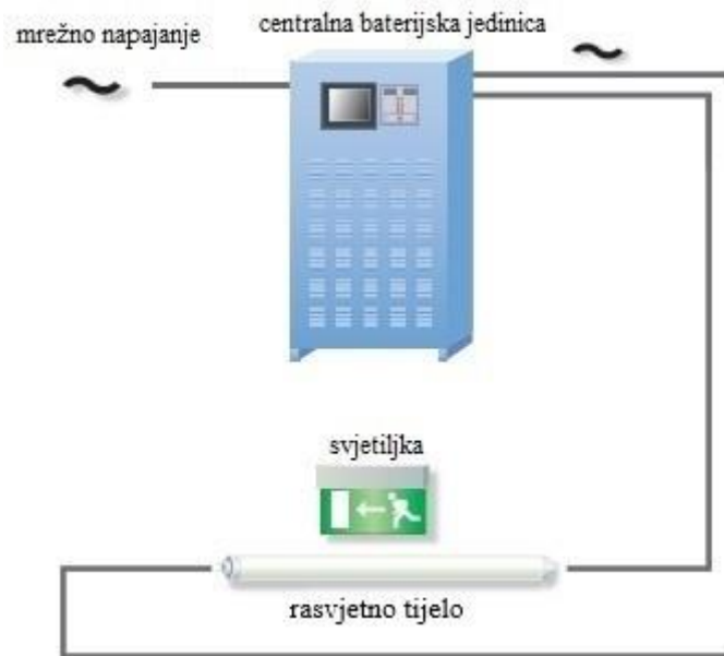
Sl.4.2. Shematski prikaz sustava s centralnim napajanjem [4]
