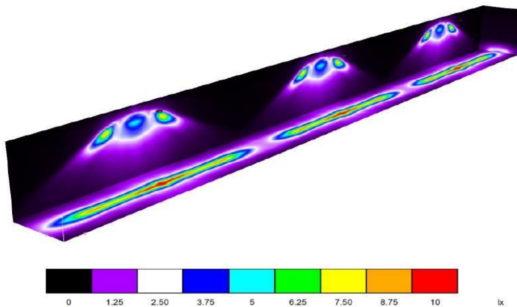
Sl. 5.9. 3-D prikaz prostorije s karakterističnim svjetilkama
