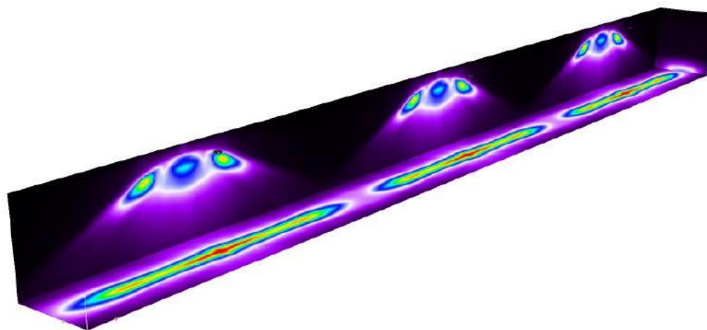
Sl. 5.9. 3-D prikaz prostorije s karakterističnim svjetiljkama
