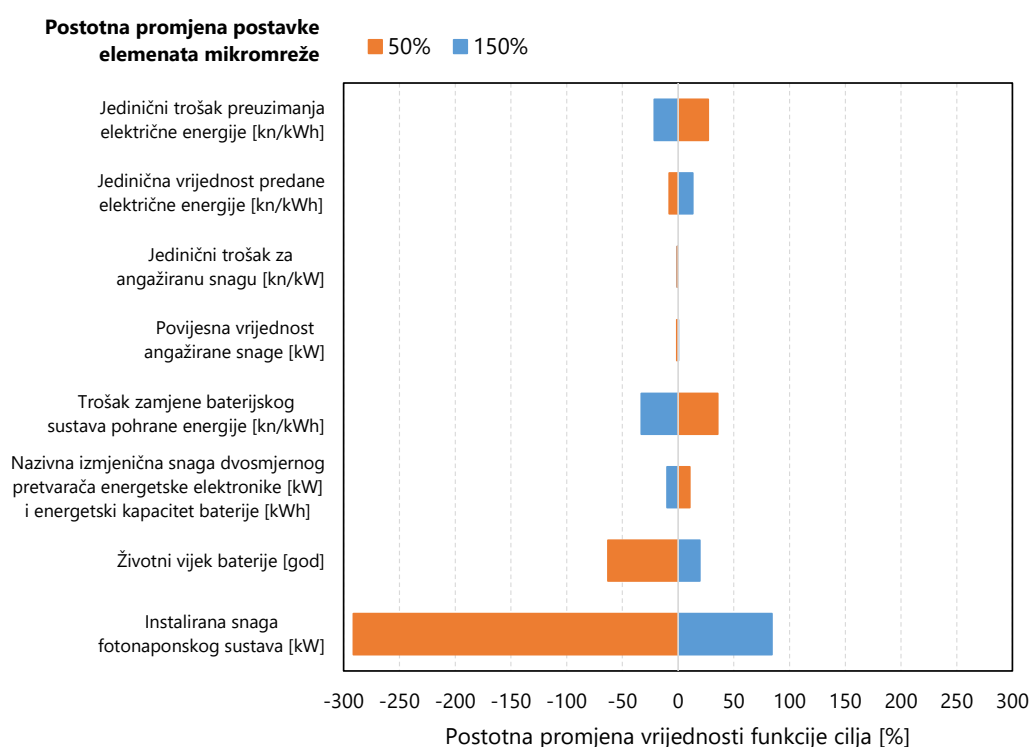
Slika 5.38: Analiza osjetljivosti vrijednosti funkcije cilja na postavke elementa mreže (mjesto priključka mikromreže na nadređenu elektroenergetsku mrežu), postavke baterijskog sustava pohrane energije i postavke fotonaponskog sustava
