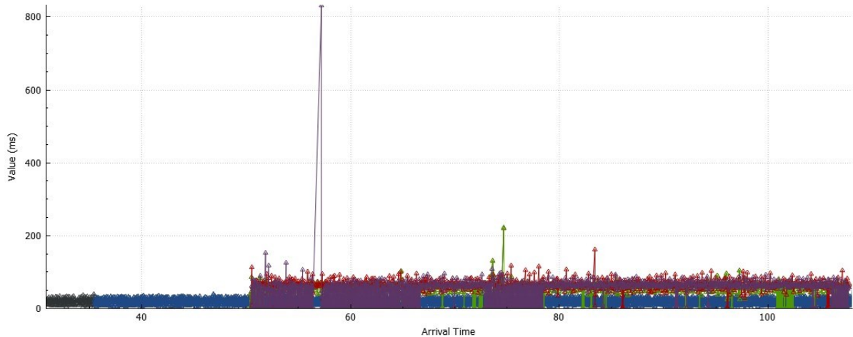
Slika 59. "Stream Delta" audio i video signala: pozivatelj-SIP poslužitelj
