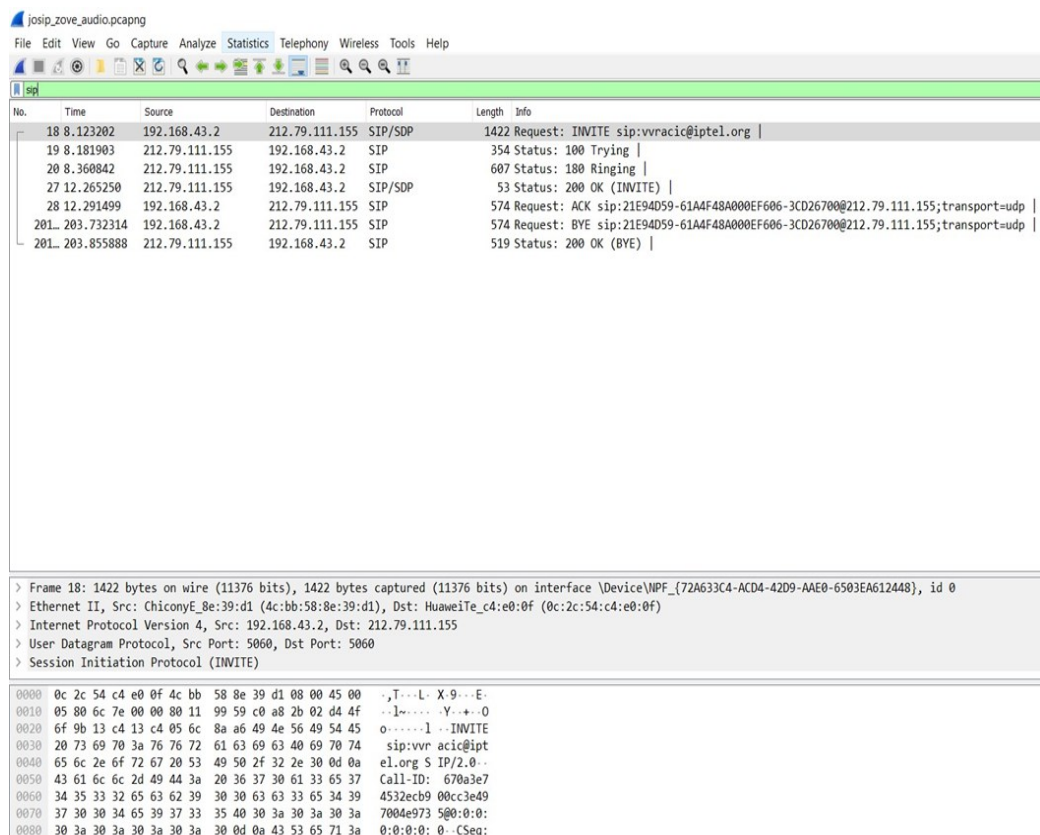
Slika 16. Rezultat filtriranja SIP protokola
