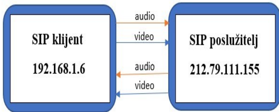
Slika 45. Pojednostavljeni prikaz razmjene RTP paketa
